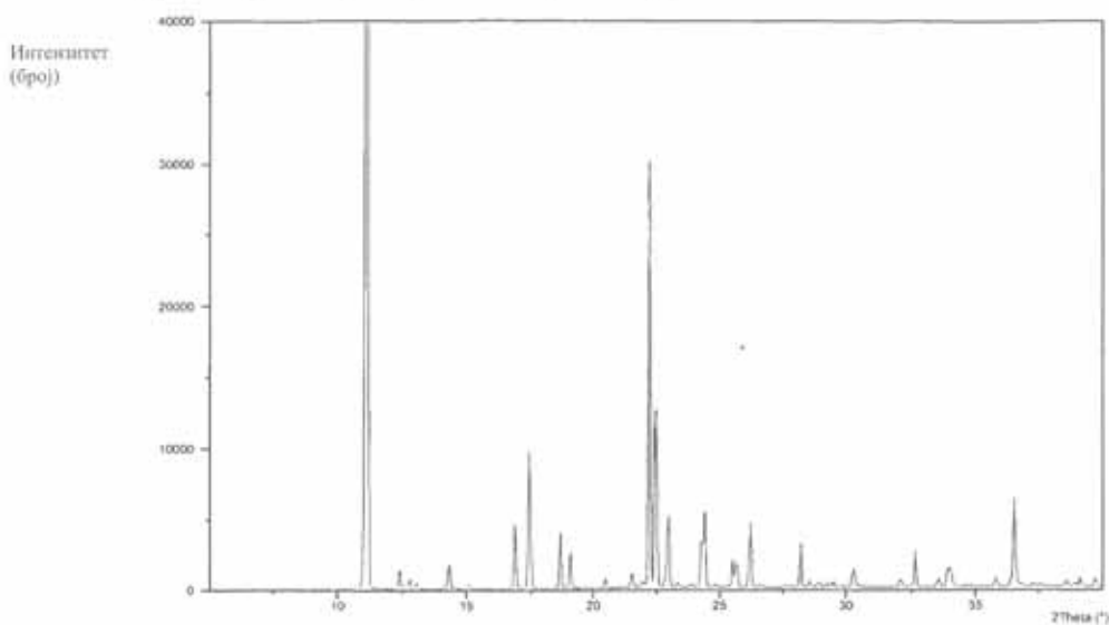
Дифрактограм на прав со рентгенски зраци без кристална база
